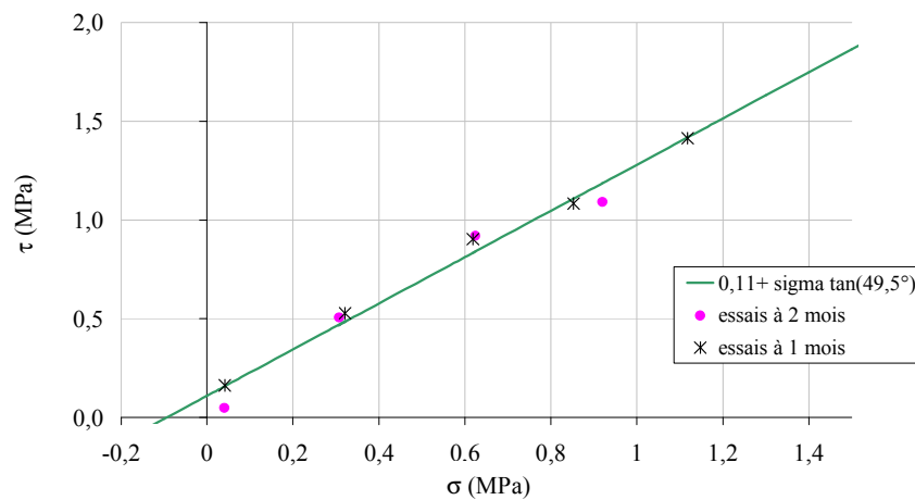
Figure 69 - Essais à l'aide de la boîte de Casagrande. Courbe intrinsèque de l'interface brique/mortier.
