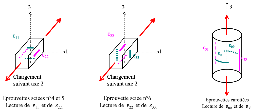
Figure 41 - Position des jauges extensométriques sur les éprouvettes en brique.
