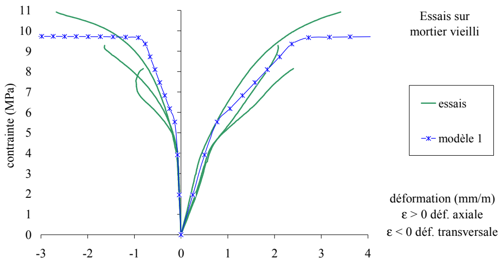
Figure 64 - Modélisation du comportement du mortier vieilli.
