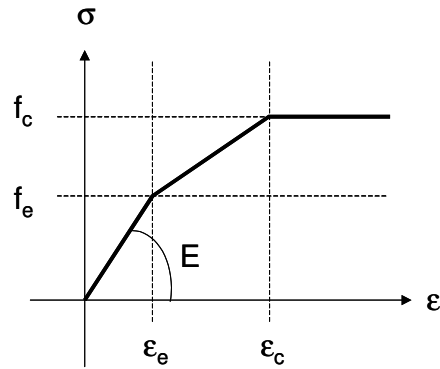
Figure 86 - Modèle de comportement adopté pour les matériaux des ponts de l'ancienne ligne de chemin de fer.
