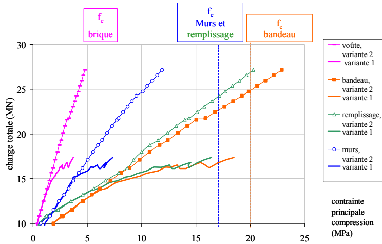
Figure 113 - Calcul variante 2. Comparaison avec la variante 1.
