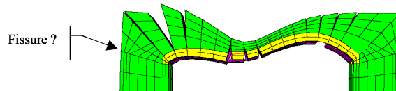
Figure 94 - Position éventuelle de fissures à l'arrière de la culée gauche.
