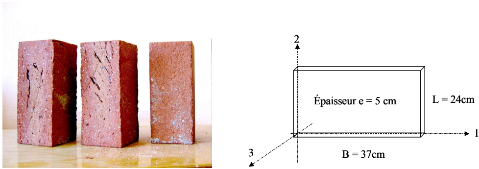
Figure 39 - A gauche : photo de briques sciées. A droite : notation des axes.
