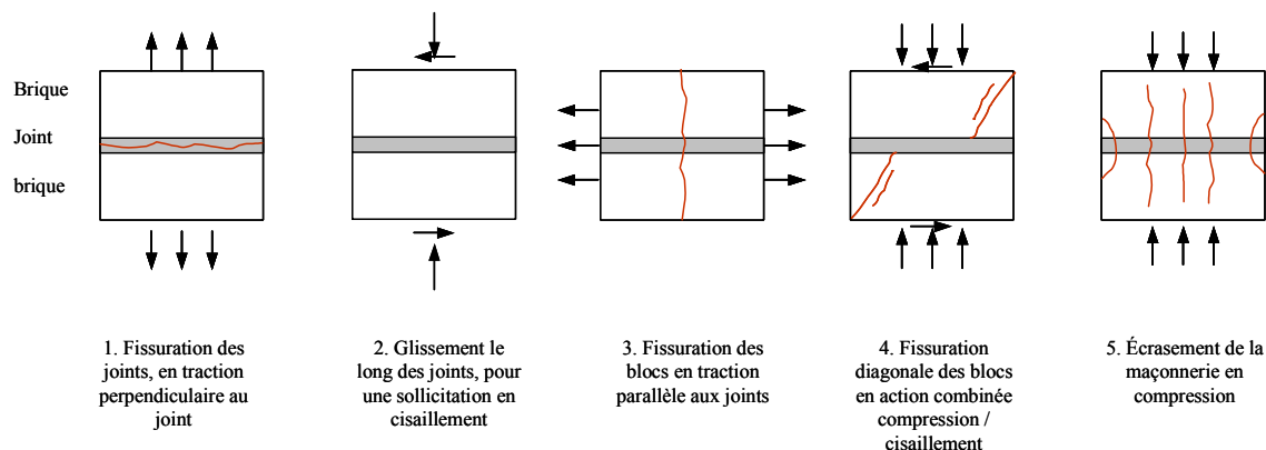
Figure 16 - Mécanismes de base de rupture d'un joint de mortier entre deux blocs 65 .
