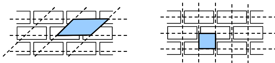
Figure 18 - Cellule de base proposée par Pegon et Antoine en 1997 (à gauche), et par A. Zucchini et P.B. Lourenço en 2004 (à droite).
