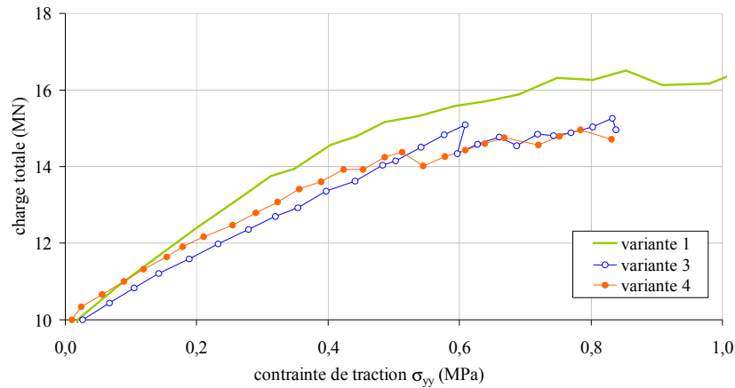
Figure 117 - Calculs variantes 3, 4 et 5 : contraintes de traction en intrados, sous l'essieu avant.
