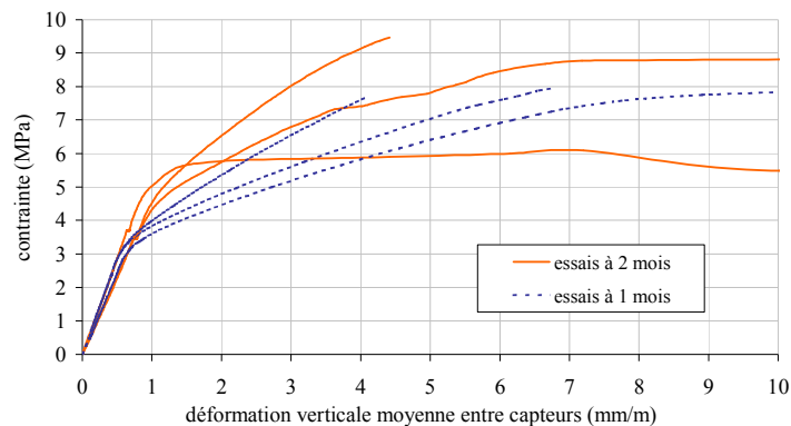
Figure 50 - Essais sur sandwichs. Variation contrainte – déformation moyenne entre capteurs, à 1 mois et 2 mois.
