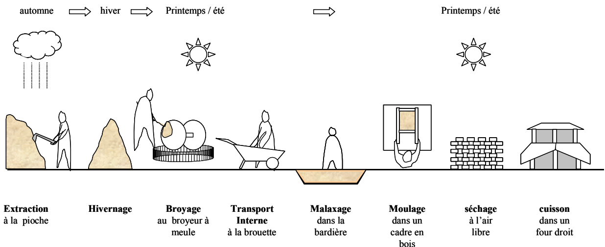
Figure 4 - Fabrication saisonnière des briques jusqu'au XIX e siècle, en Midi-Pyrénées.
