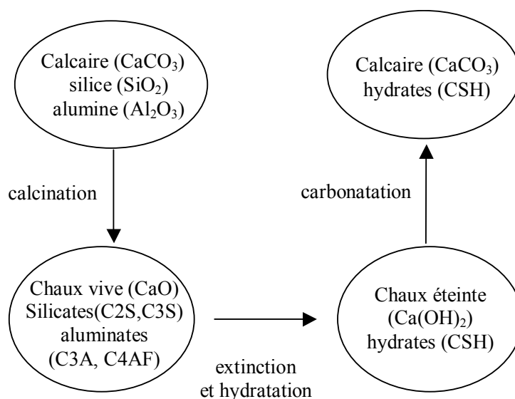
Figure 7 - Prise de la chaux hydraulique.
