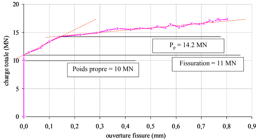
Figure 93 - Calcul de base : ouverture des fissures sous l'essieu avant.
