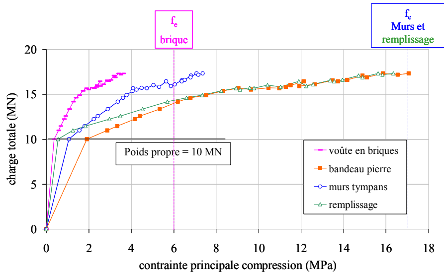
Figure 98 - Calcul de base : compression principale dans les matériaux.
