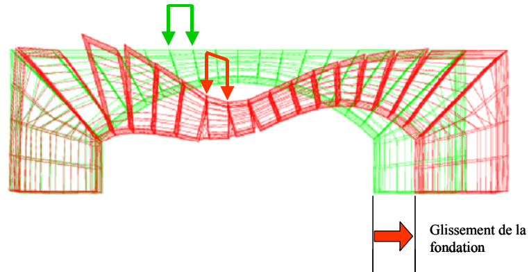
Figure 91 - Déformée du pont, en rouge. Configuration initiale en vert.
