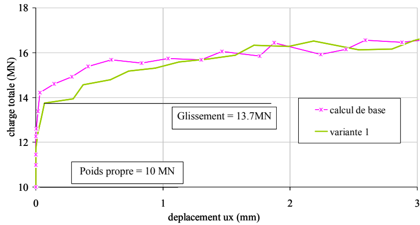
Figure 108 - Calcul variante 1. Glissement sur le sol de fondation.
