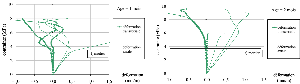
Figure 51- Essais sur sandwichs, comportement des joints de mortier.
