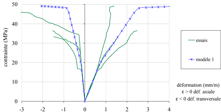
Figure 74 - Comportement de la pierre. Essais et modèle théorique.
