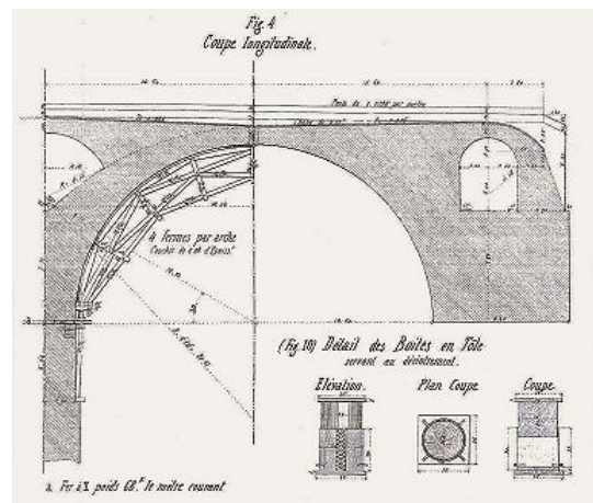
Figure 2 - Cintre et boîtes à sable du Viaduc d'Albi; d'après archives SNCF.
