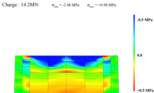
Figure 103 - Contraintes \sigma_{yy} entre les essieux du tandem pour P = 14.2\text{MN} .
