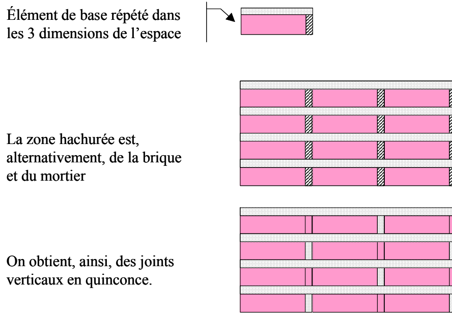
Figure 47 - Construction numérique d'un mur en brique à l'aide d'un élément de base répété en translation.
