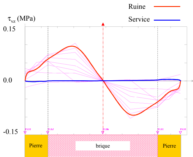
Figure 107 - Contraintes de cisaillement \tau_{xy} le long de l'intrados, sous l'essieu avant du tandem.
