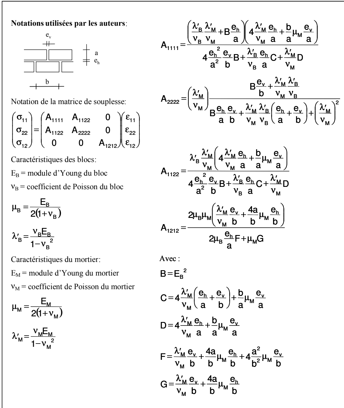
Figure 20 – Homogénéisation analytique en 2D. Formulation de Cecchi et Sab. 2002.
