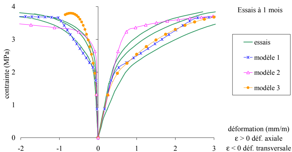
Figure 58 - Modélisation du comportement du mortier. Comparaison avec les 3 modèles retenus à 1 mois.
