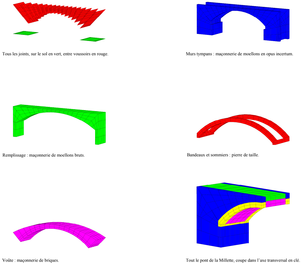
Figure 88 - Modélisation du pont de la Millette avec 16 voussoirs. Répartition des 4 maçonneries et des joints.
