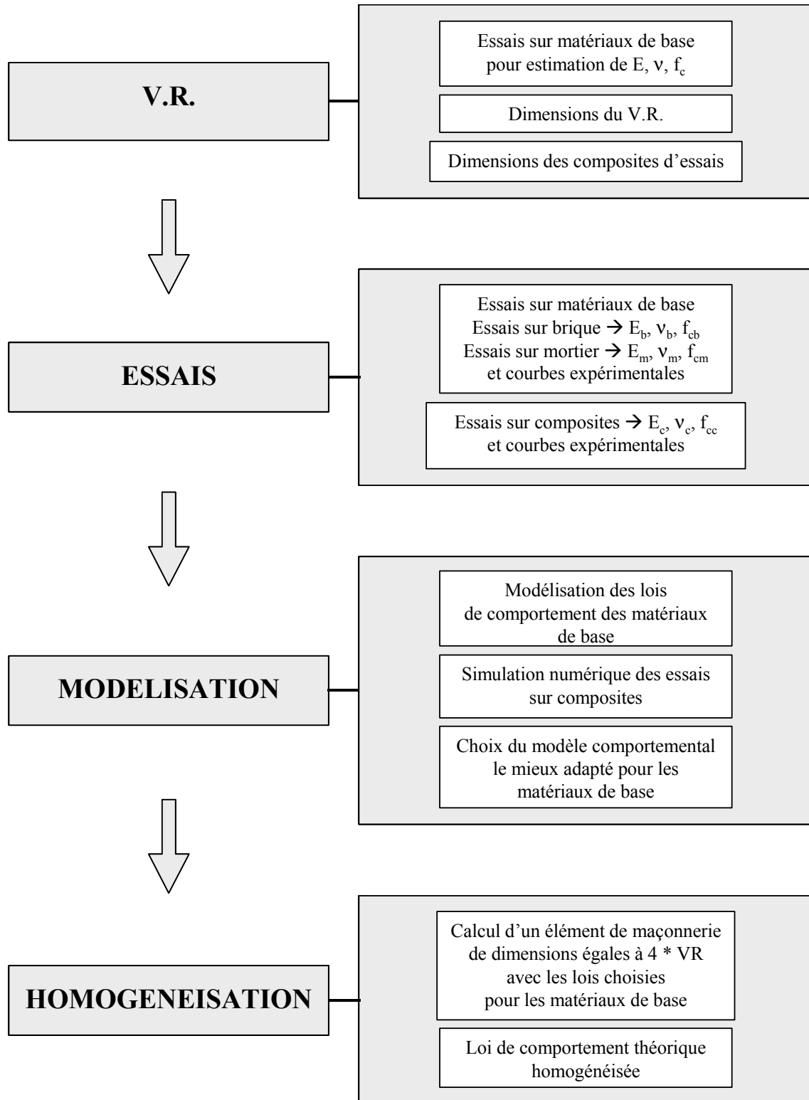
Figure 56 - Méthode d'homogénéisation expérimentale et numérique.
