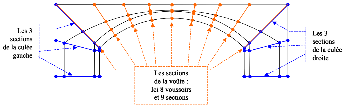
Figure 82 - Maillage du pont. Découpage du pont en sections. Dessin pour 8 voussoirs.
