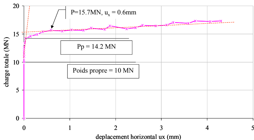
Figure 90 - Calcul de base : glissement de la fondation sur le sol.
