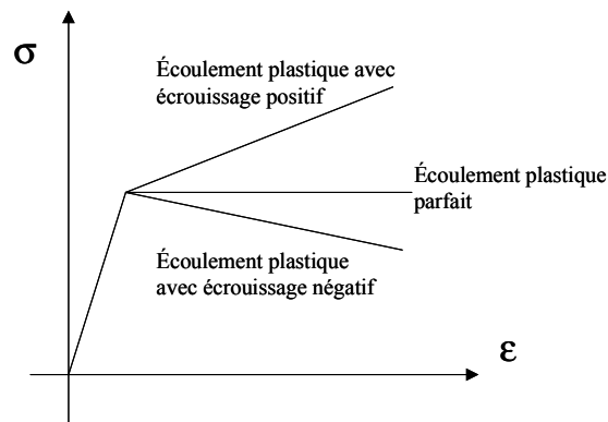
Figure 14 - Ecrouissage d'un matériau sous chargement monoaxial.
