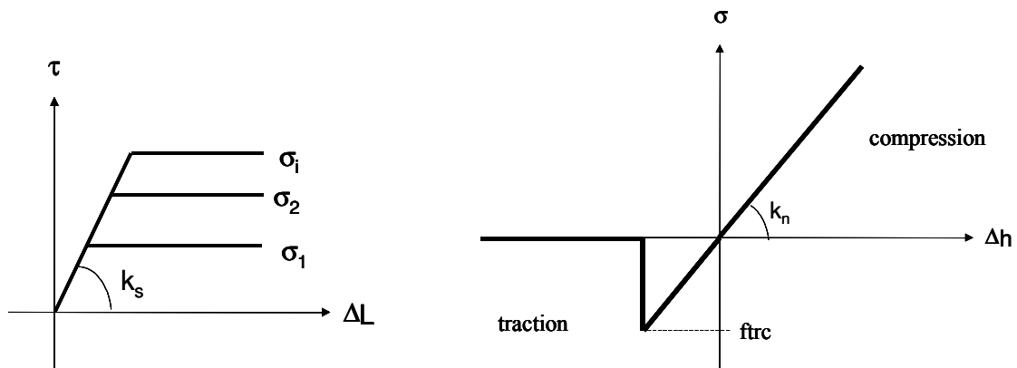
Figure 70 - Modèle de joint. A gauche : comportement en cisaillement. A droite : comportement en traction / compression.
