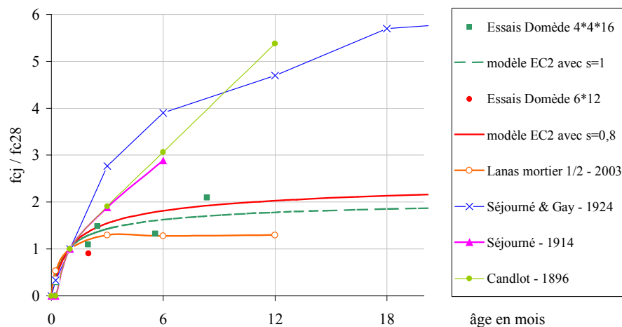
Figure 44 - Loi de comportement du mortier de chaux. Comparaison des essais réalisés aujourd'hui et des valeurs bibliographiques.
