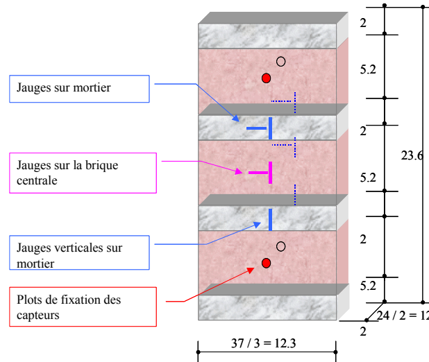
Figure 46 - Schéma des "sandwiches".
