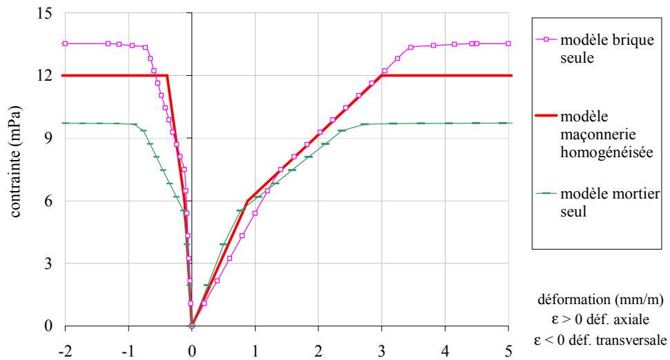
Figure 65 - Modélisation de la maçonnerie de brique. Comparaison avec les matériaux de base.
