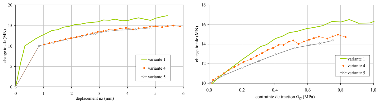
Figure 120 - Comparaison calculs variantes 4 et 5. Déplacement vertical sous essieux et traction transversale.
