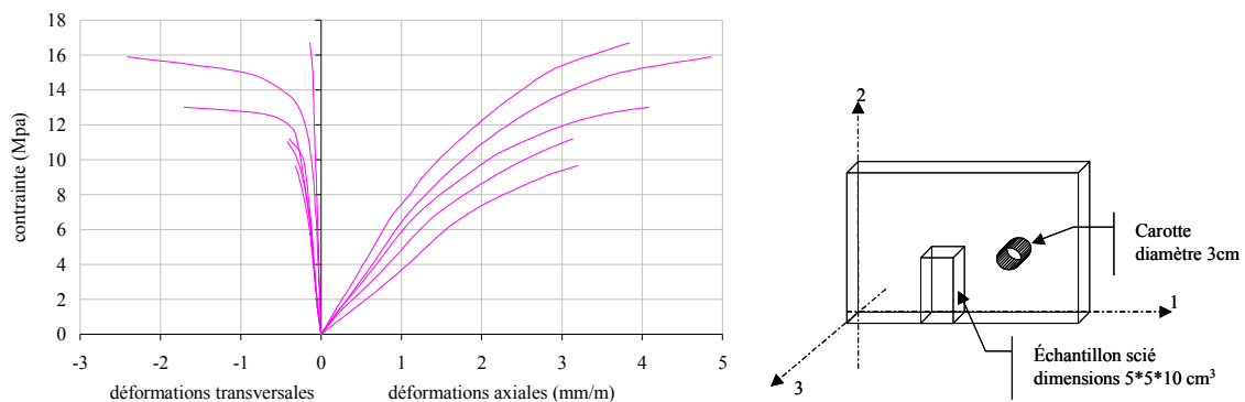
Figure 45 - Essais sur brique. Résultats des essais de compression sur carottes. Variation contrainte / déformation axiale et transversale. Dernière montée en charge.
