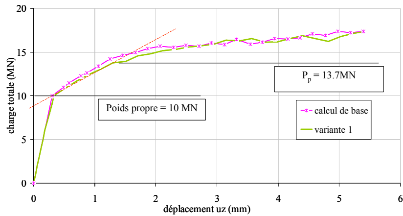
Figure 109 - Calcul variante 1. Déplacement vertical des points d'impact du tandem.
