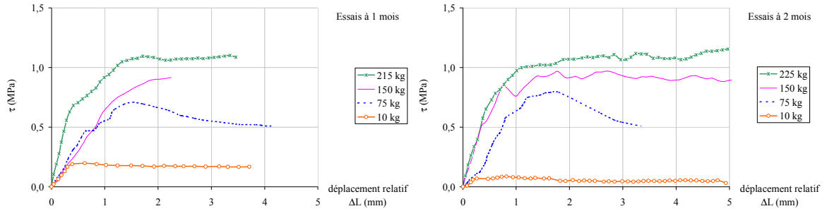
Figure 68 - Essais à l'aide de la boîte de Casagrande. Variation \tau / \Delta L à 1 mois et 2 mois.
