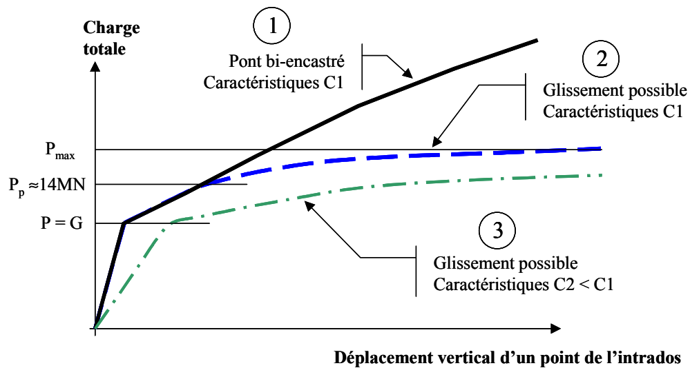
Figure 122 - Variation du déplacement vertical de l'intrados lorsque la charge appliquée augmente.
