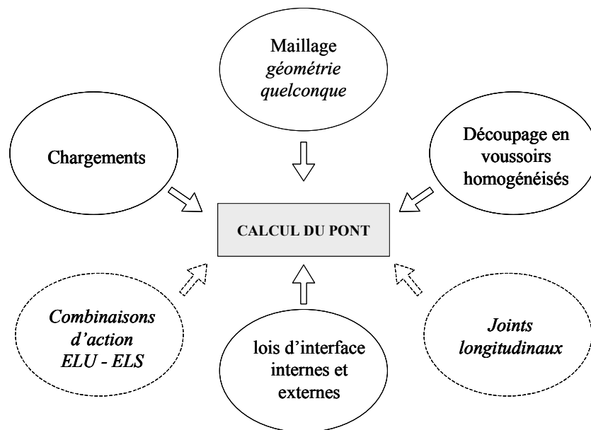
Figure 127 – 4 ème étape : Calcul du pont.
