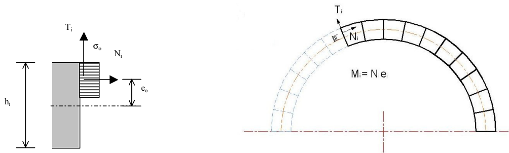
Figure 13 - Méthode de calcul du SETRA, programme VOUTE. Equilibre des voussoirs, 1982.
