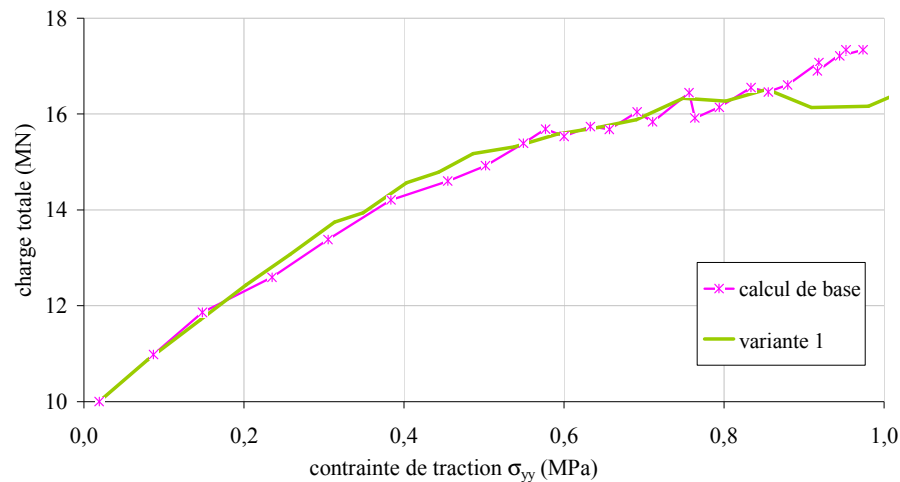
Figure 111 - Calcul variante 1. Contrainte de traction en intrados, sous l'essieu avant.
