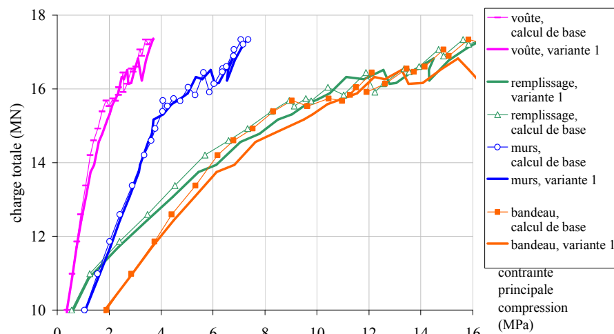
Figure 112 - Calcul variante 1. Compressions principales dans les matériaux.
