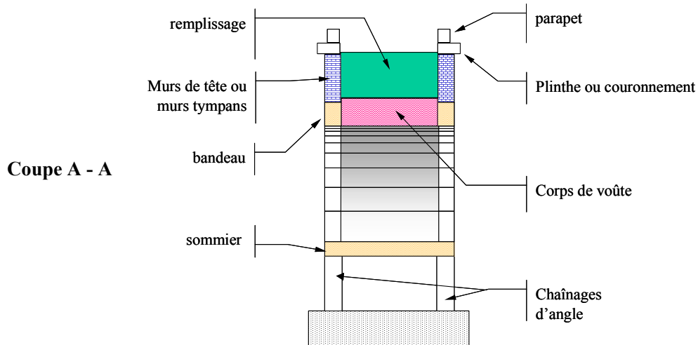
Figure 1 - Terminologie des ponts en maçonnerie.
