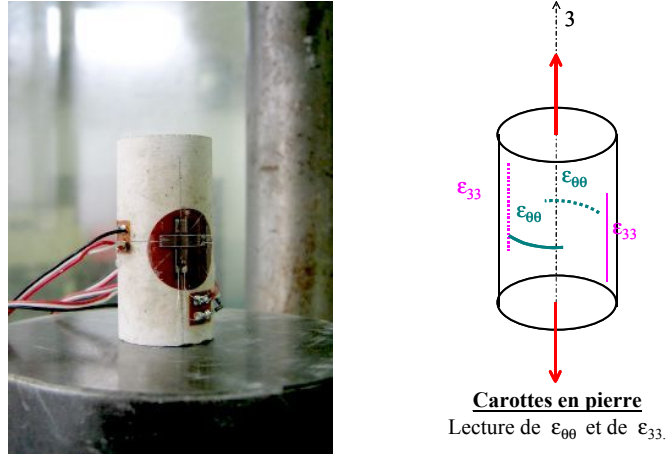
Figure 72 - Echantillons de pierre pour essais mécaniques.
