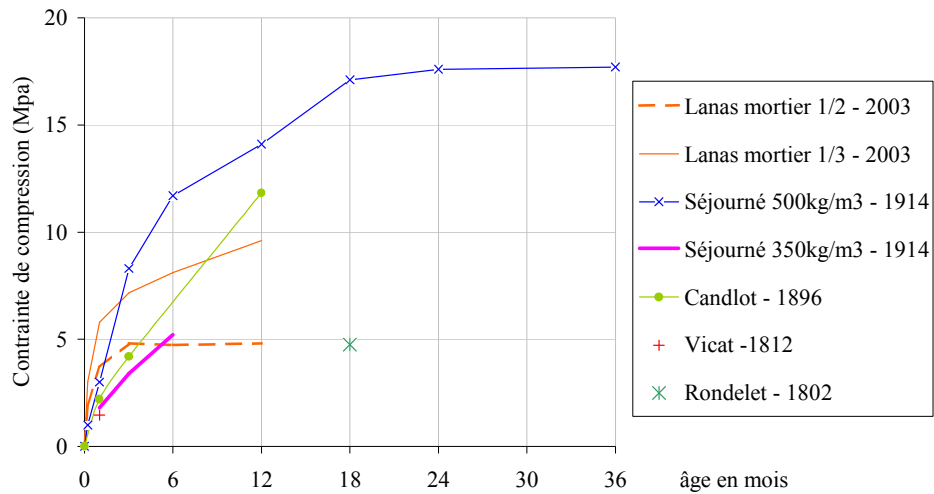
Figure 9 - Résistance du mortier avec l'âge selon différents auteurs.
