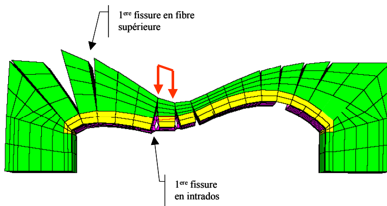
Figure 92 - Déformée du pont et fissuration au dernier pas de calcul.
