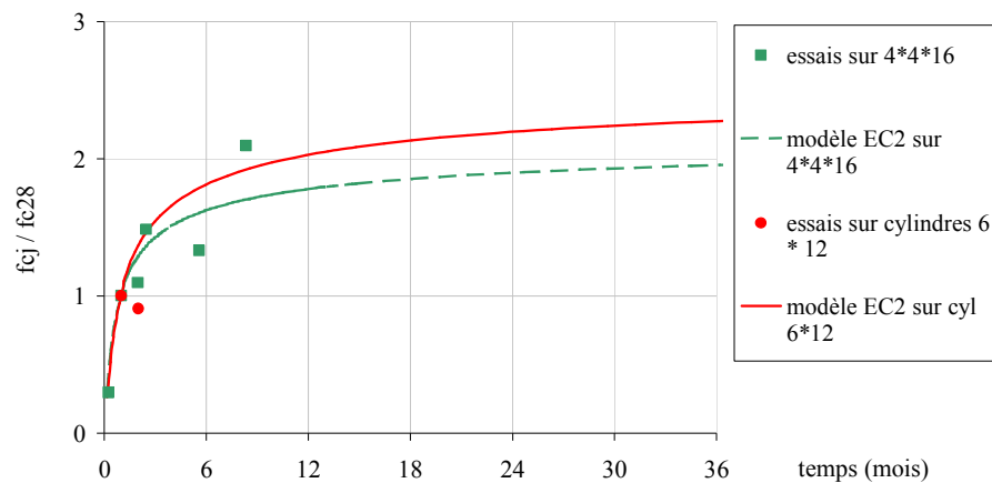
Figure 43 - Comportement du mortier de chaux en fonction du temps. Essais et modèle.
