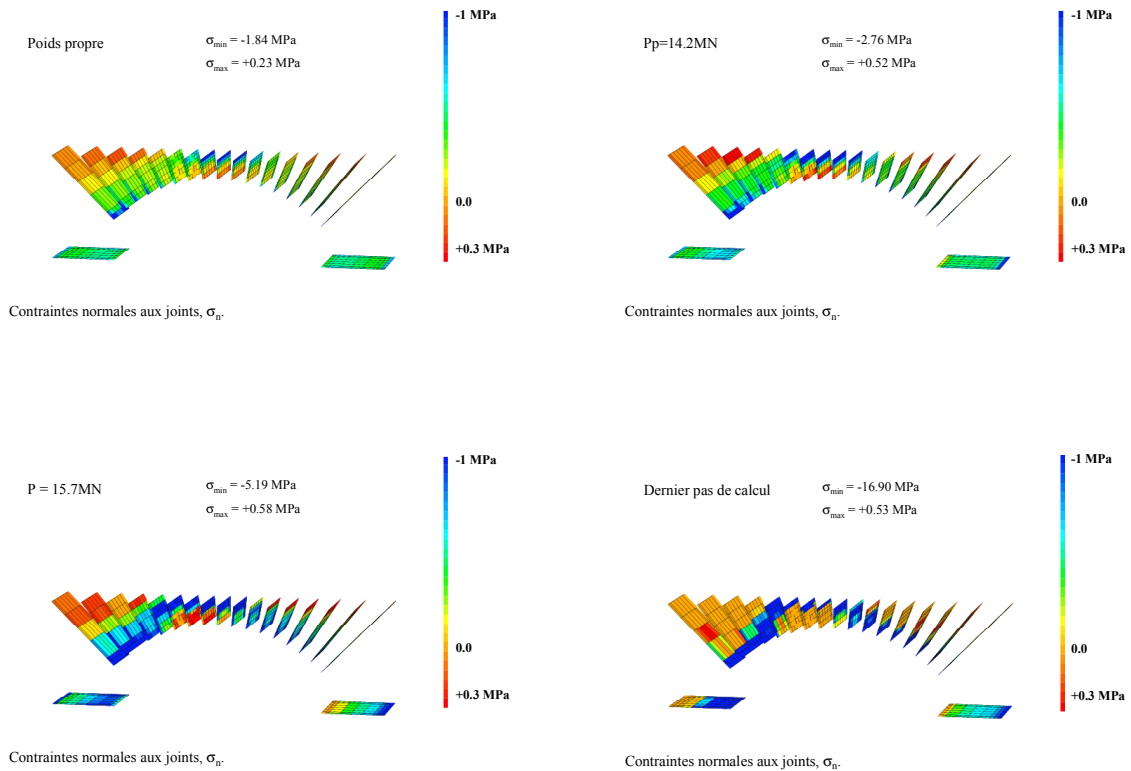
Figure 100 - Contraintes normales aux joints. La compression dépasse (en valeur absolue) 1 MPa dans les zones bleues. La traction dépasse 0.3MPa dans les zones rouges.
