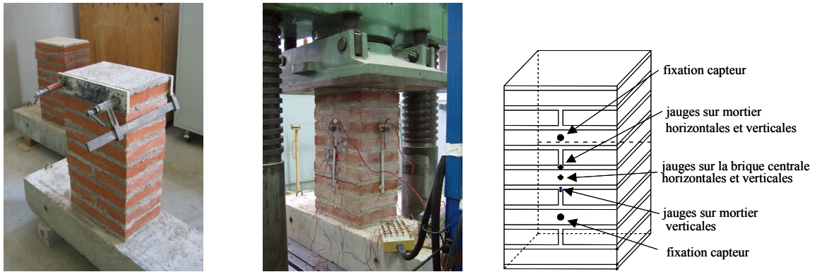
Figure 48 - Photo des murets, avant et pendant l'essai. Schéma de la position des jauges et des capteurs.
