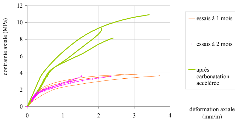
Figure 42 - Essais sur mortier de chaux jeune et vieilli, éprouvettes cylindriques 6*12, variation contrainte – déformation axiale.
