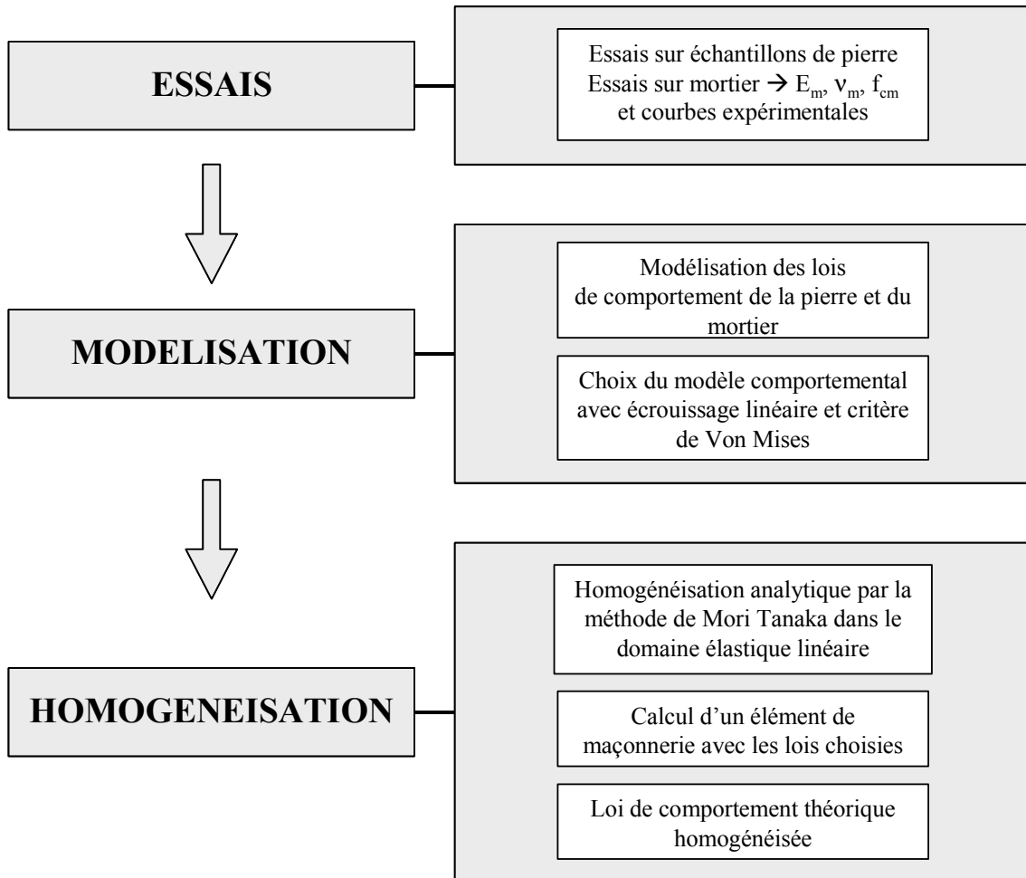
Figure 76 - Méthode d'homogénéisation de la maçonnerie de moellons en opus incertum.
