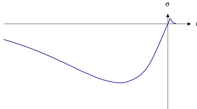
Figure 15 - Modèle de Mazars, comportement unidirectionnel en traction et en compression.
