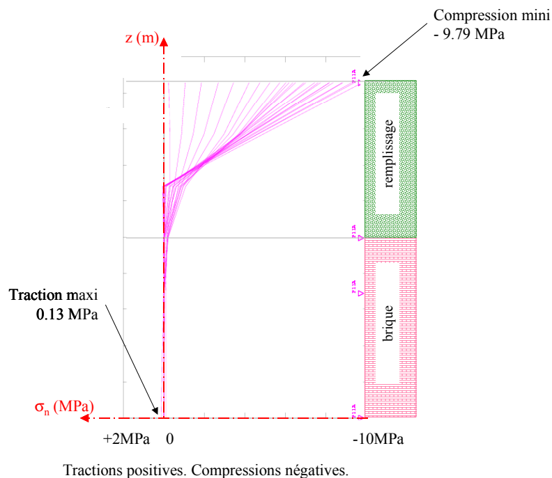
Figure 99 - Contraintes normales au joint situé sous l'essieu arrière du tandem. Variation de \sigma_n le long de l'axe vertical du pont.
