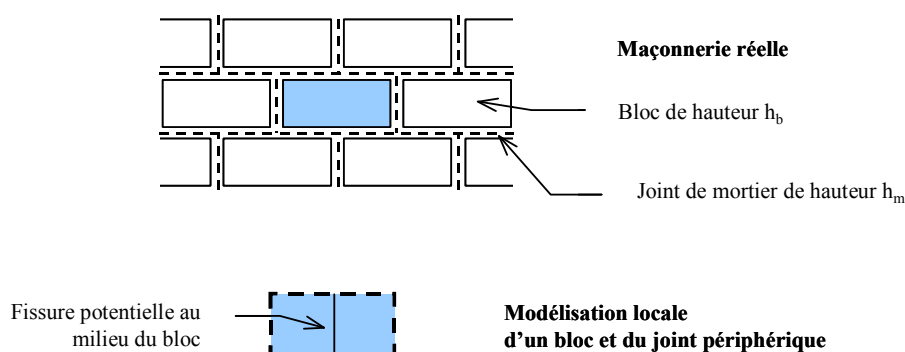
Figure 17 - Principe de la modélisation locale simplifiée selon Lourenço 71 .
