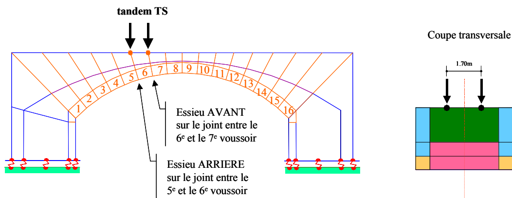
Figure 87 - Chargement du pont, position du tandem sur l'ouvrage.
