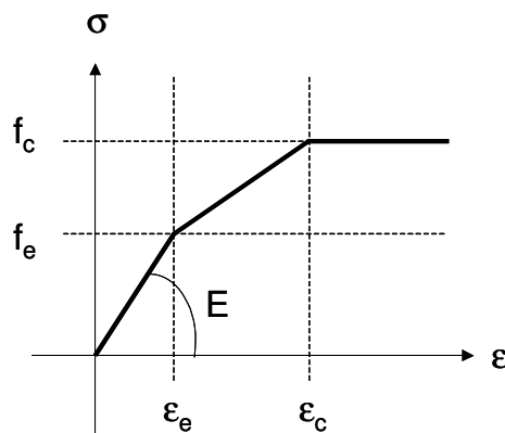
Figure 57 - Modèle 1 : modèle élasto-plastique, avec critère de plasticité de Von Mises.
