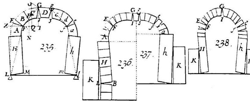
Figure 11 - Mécanismes de ruine des voûtes, d'après Amédée Frézier, 1739.
