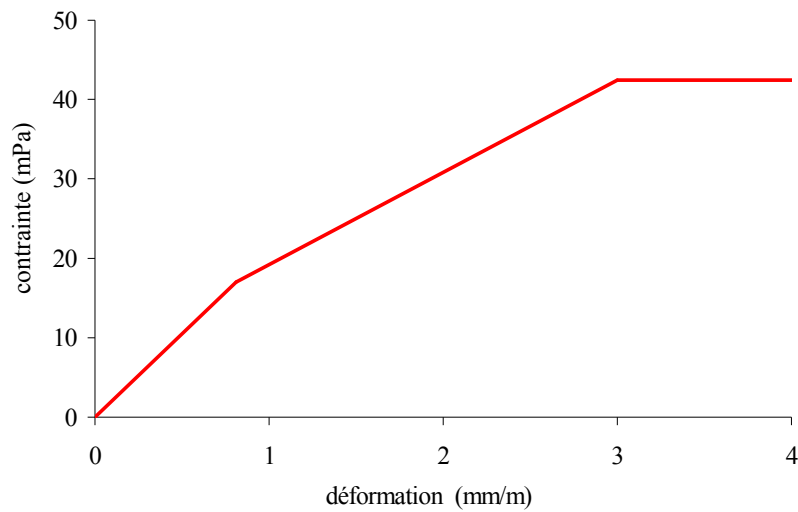
Figure 75 - Modélisation du comportement des maçonneries de moellons.
