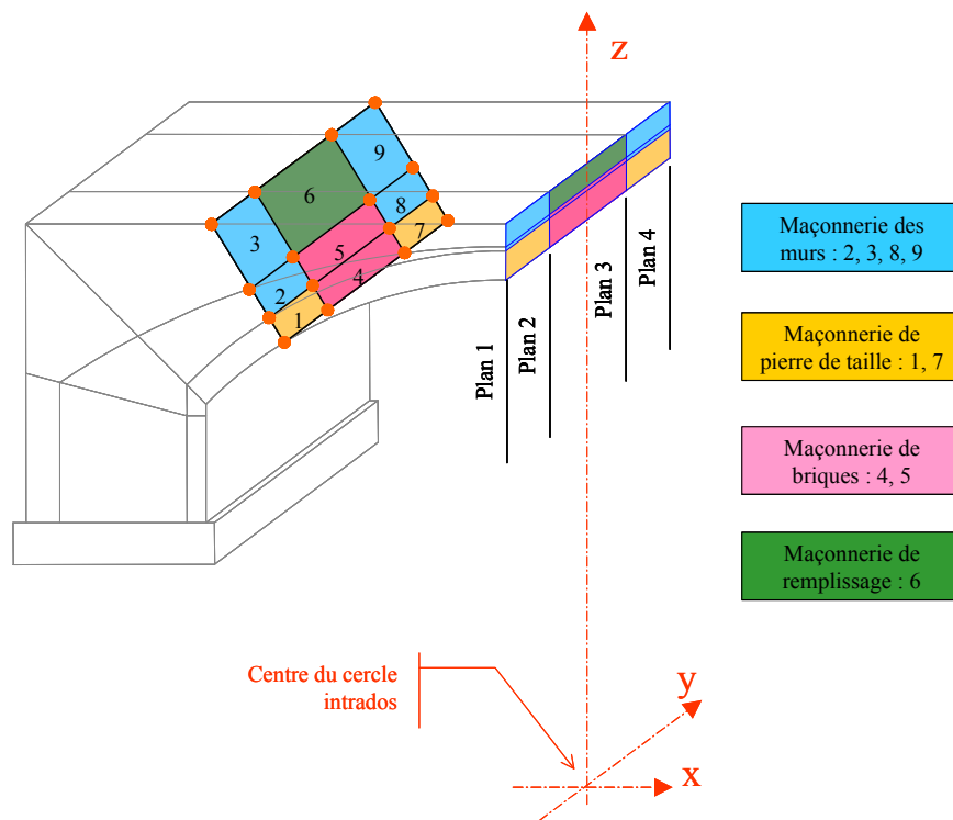
Figure 83 - Maillage du pont. Découpage des sections en 9 surfaces élémentaires. Tous les points sont sur 4 plans parallèles.
