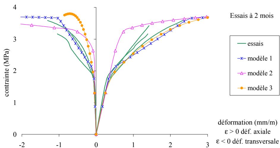
Figure 59 - Modélisation du comportement du mortier. Comparaison avec les 3 modèles retenus à 2 mois.
