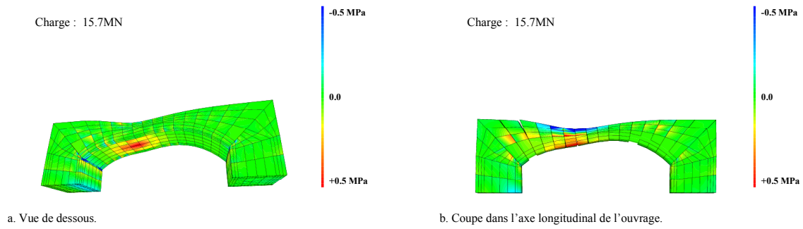
Figure 101 - Tractions principales dans le pont de la Millette pour P = 15.7\text{MN} . Les contraintes de traction dépassent 0.5\text{MPa} dans les zones rouges.
