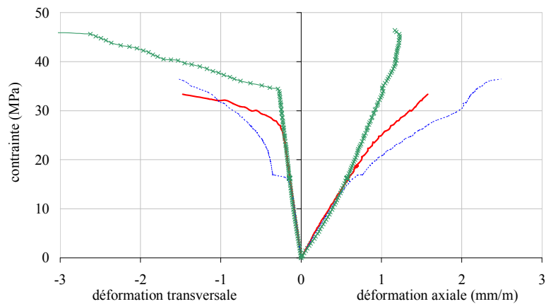
Figure 73 - Comportement des pierres. Résultats des essais.
