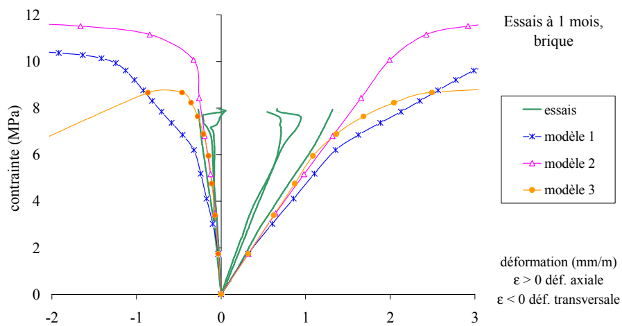
Figure 61 - Modélisation du comportement des sandwiches à 1 mois. Comparaison des 3 modèles et des essais. a : en haut, enregistrement des capteurs ; b : au milieu : enregistrement des jauges collées sur les joints de mortier ; c : en bas , enregistrement des jauges collées sur les briques.
