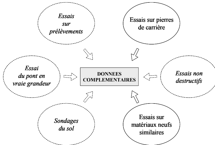
Figure 125 – 2 ème étape : recueil des données complémentaires.
