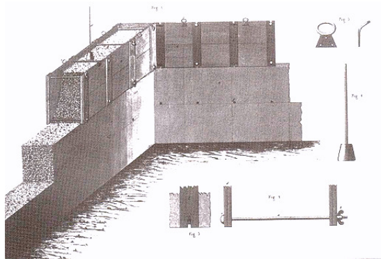
Figure 10 - Système Lebrun de construction en béton, 1832. D'après A. Guillerme, Bâtir la ville , p. 176.
