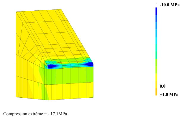
Figure 96 - Compressions principales sur la culée gauche, dernier pas de calcul.
