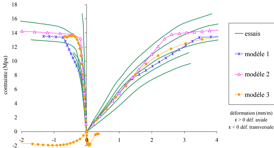
Figure 60 - Modélisation du comportement des briques. Comparaison avec les 3 modèles retenus.
