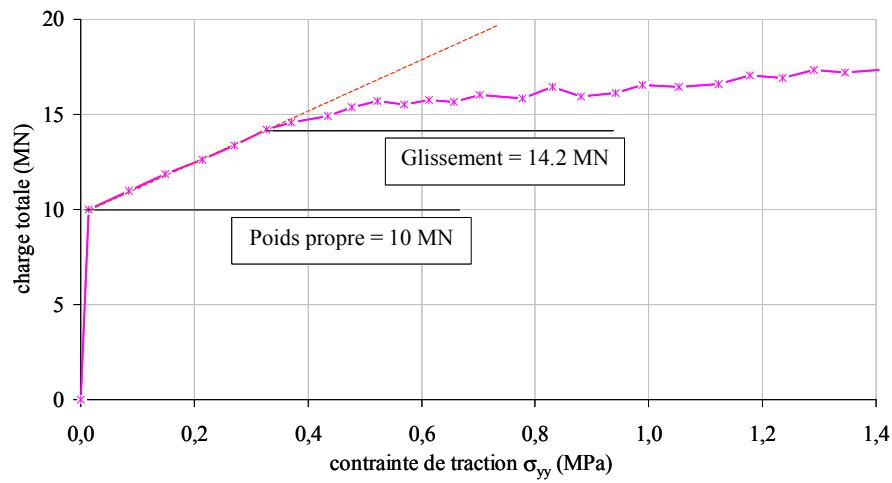
Figure 102 - Variation de la traction maximale \sigma_{yy} , dans l'axe du pont, sous l'essieu avant.
