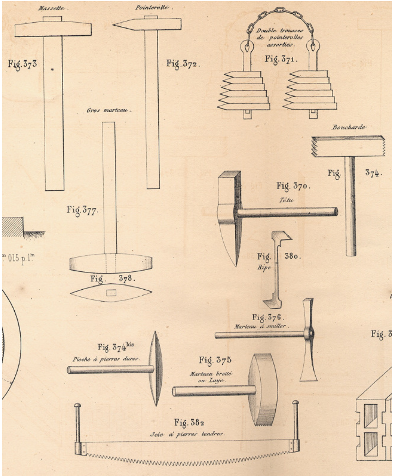
Figure 32 - Les outils du tailleur de pierre, d'après Debaue, Manuel de l'ingénieur des Ponts et Chaussées, Paris : Dunod, 1873, planche 48.
