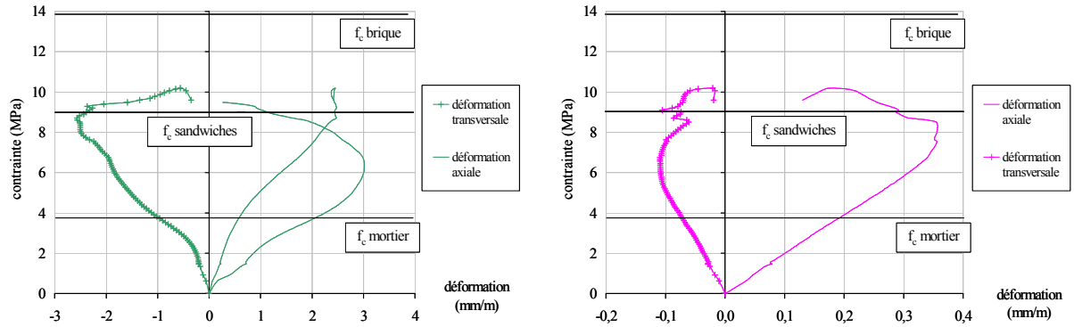
Figure 55 - Essais sur muret. Variation contrainte – déformations axiales et transversales des joints de mortier et des briques.
