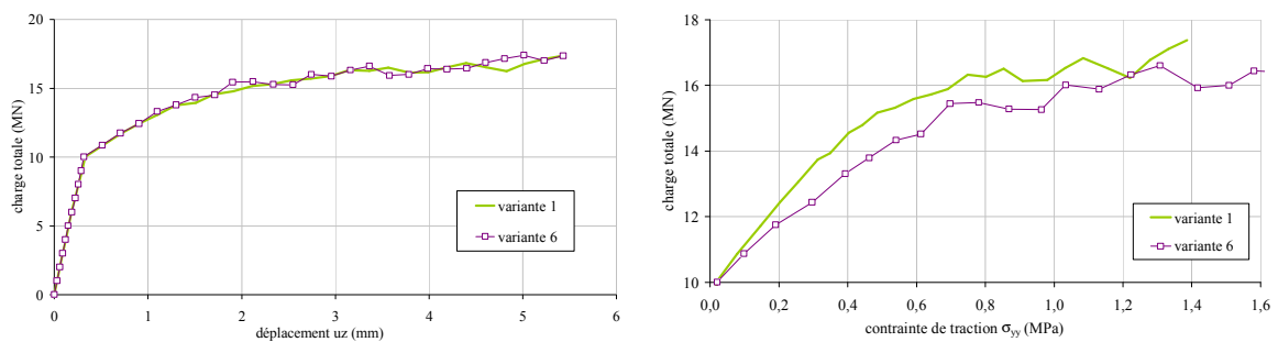
Figure 121 - Comparaison des variantes 1 et 6. Déplacements verticaux et contraintes de traction \sigma_{yy} .
