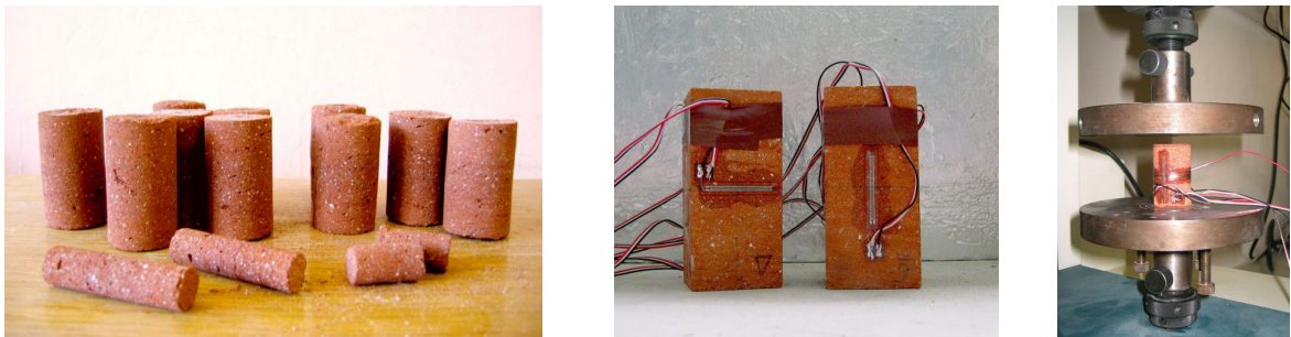
Figure 40 - A gauche : photo des carottes de brique. Au milieu et à droite : éprouvettes équipées de jauges, avant essais.
