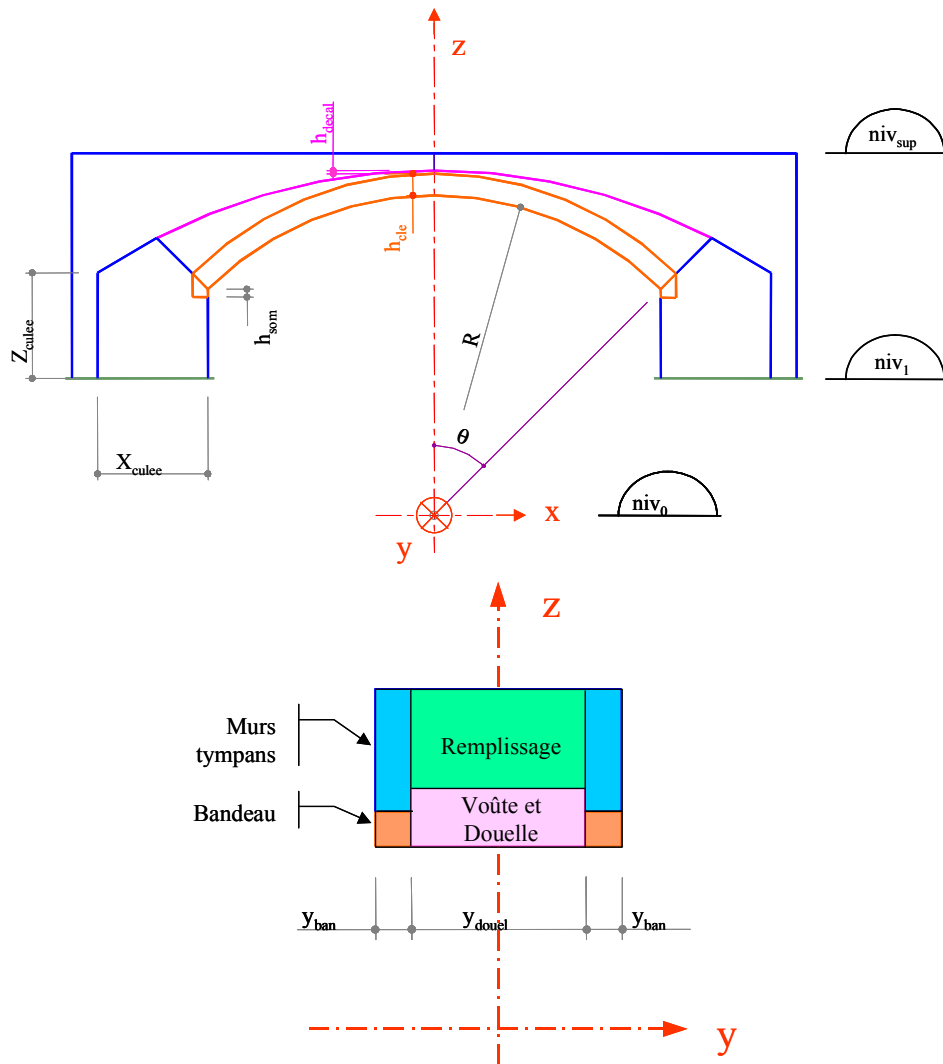
Figure 81 - Calcul du pont de la Millette, géométrie du modèle.
