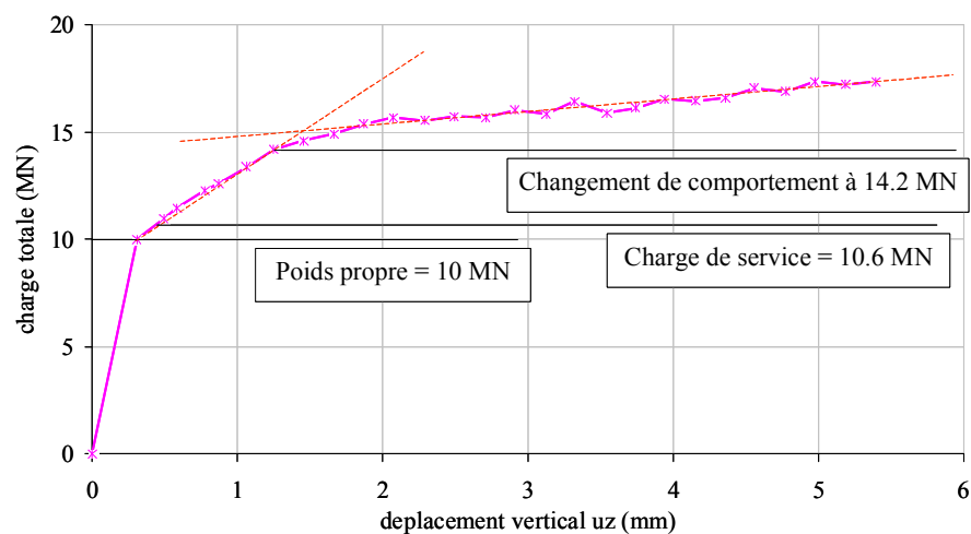
Figure 89 - Calcul de base : déplacement vertical des points d'impact des essieux.
