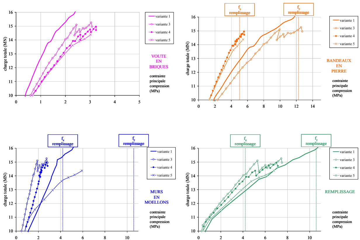
Figure 118 - Calculs variantes 1, 3, 4 et 5 : compressions extrêmes (en valeur absolue) dans les maçonneries.
