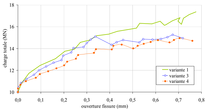
Figure 116 - Calculs variantes 3, 4 et 5 : ouverture des fissures sous l'essieu avant.
