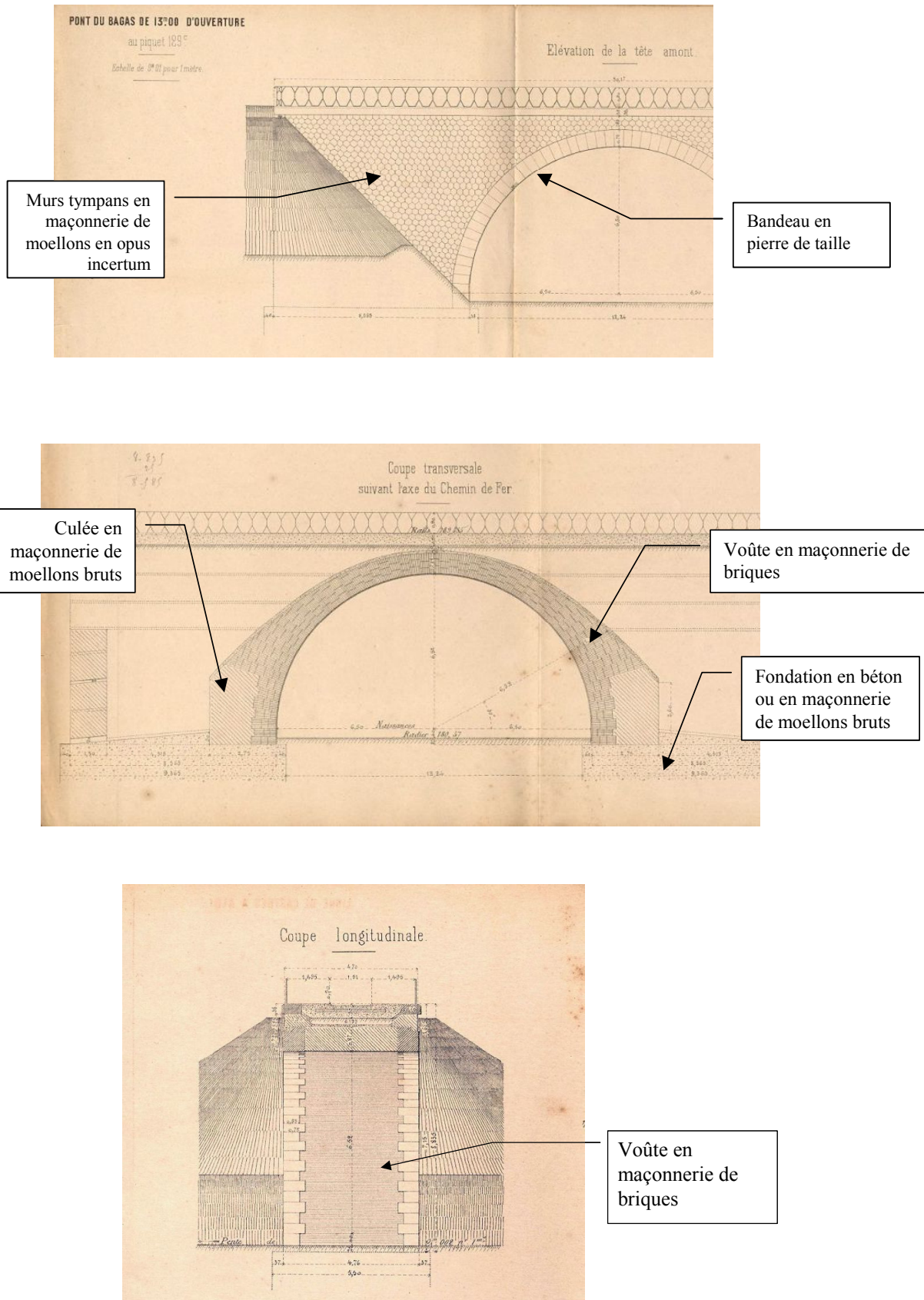
Figure 29 - Répartition des matériaux dans les ponts en maçonneries. Plans du pont du Bagas. Archives SNCF.
