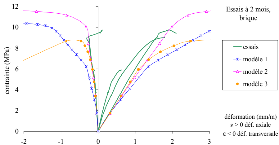
Figure 62 - Modélisation du comportement des sandwiches à 2 mois. Comparaison des 3 modèles et des essais.
