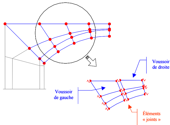
Figure 85 - Principe du découpage de la voûte en voussoirs liés par des joints. Dessin éclaté, pour 8 voussoirs.
