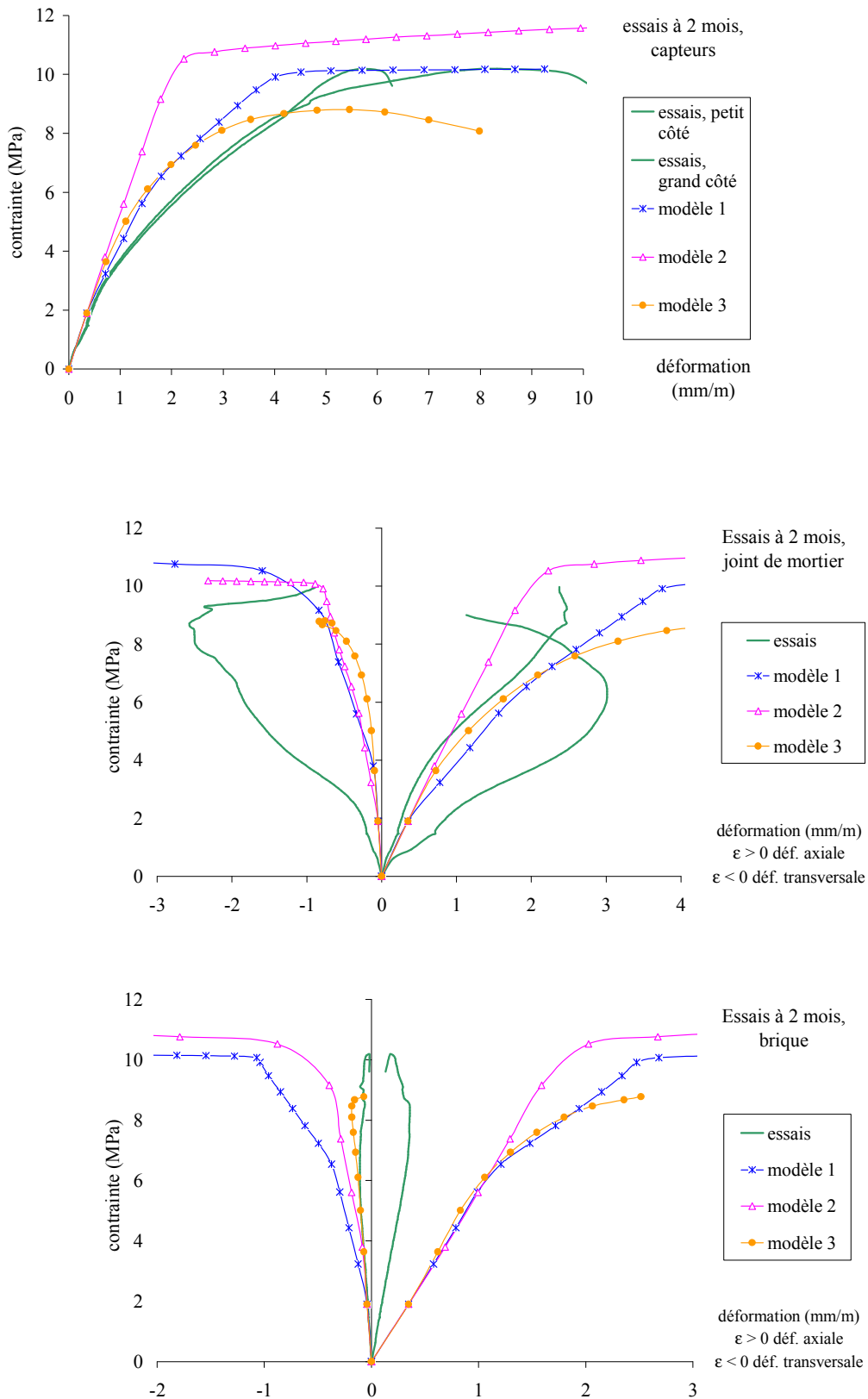
Figure 63 - Modélisation du comportement des murets à 2 mois. Comparaison des 3 modèles et des essais. a : en haut, enregistrement des capteurs ; b : au milieu : enregistrement des jauges collées sur les joints de mortier ; c : en bas, enregistrement des jauges collées sur les briques.
