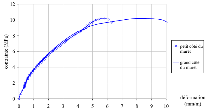
Figure 54 - Essais sur muret. Variation contrainte – déformation moyenne entre capteurs.
