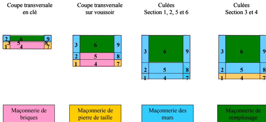
Figure 84 - Modélisation du pont. Position des 4 maçonneries homogénéisées.
