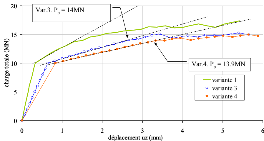
Figure 114 - Calculs variantes 3, 4 et 5 : déplacement vertical du point d'impact du tandem.
