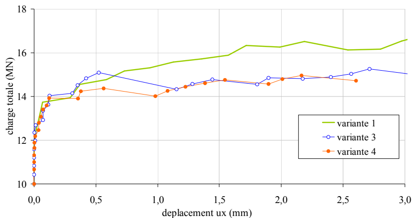
Figure 115 - Calculs variantes 3, 4 et 5 : glissement sur le sol de fondation.
