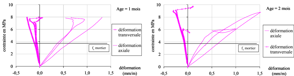
Figure 52 - Essais sur sandwichs, comportement des blocs de brique.
