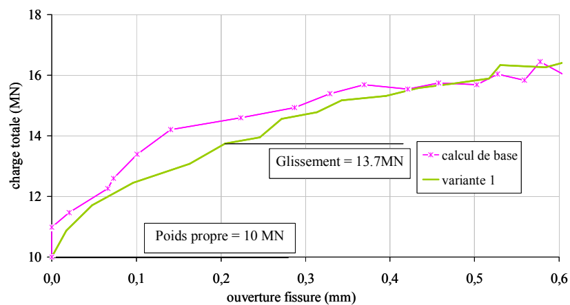
Figure 110 - Calcul variante 1. Ouverture des fissures.
