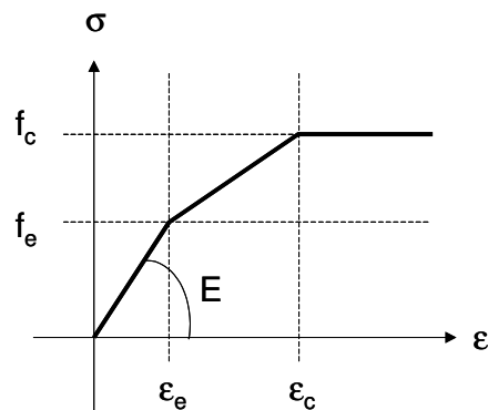
Figure 77 - Modèle de comportement adopté pour les matériaux des ponts de l'ancienne ligne de chemin de fer.
